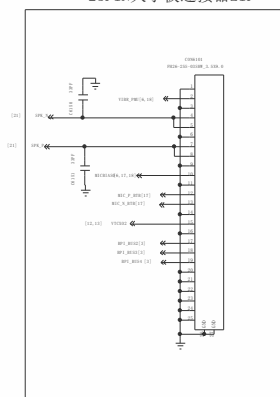
25PIN大小板连接器ZIF
